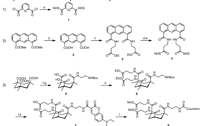
Scheme 1. Synthesis of the ready-to-use templates. a) NHS, DIEA, THF, 12h, r.t., 84%. b) LiOH, THF/MeOH/H 2 O, r.t., 4h, 90%. c) H- \beta Ala-OEt, PyBOP, DIEA, DMF, 12h, r.t., 88%. d) LiOH, THF/MeOH/H 2 O, r.t., 4h, 90%. e) NHS, WSCI•HCl, DIEA, DMF, r.t., 12h, 68%. f) Sublimation, 90%. g) H 2 N(CH 2 ) 2 NHBoc, DIEA, DMF, 6h, r.t., 88%. h) H- \beta Ala-OEt, HBTU, HOBT, DIEA, DMF, 12h, r.t., 56%. i) LiOH, THF/H 2 O 1:1, r.t., 1h, 98%. j) TFA/DCM 1:1, r.t., 30 min, 82%. k) DMACA-SE, DIEA, DMF, r.t., 12h, 45%. l) NHS, WSCI•HCl, DIEA, DMF, r.t., 12h, 84%.
